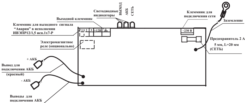
Рисунок 1– Плата источника
